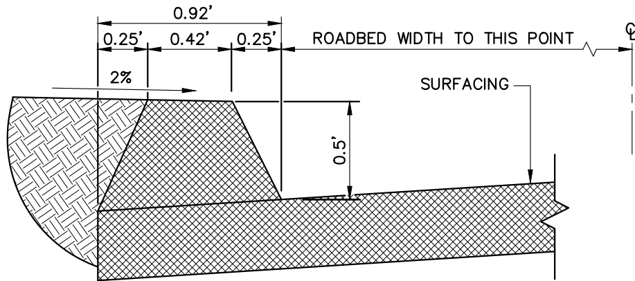
6" A.C. DIKE
